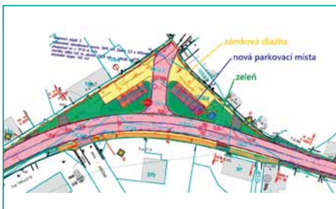
Návrh rekonstrukce křižovatky ulic – K Cihelně, K Cestkám a Branžežská
