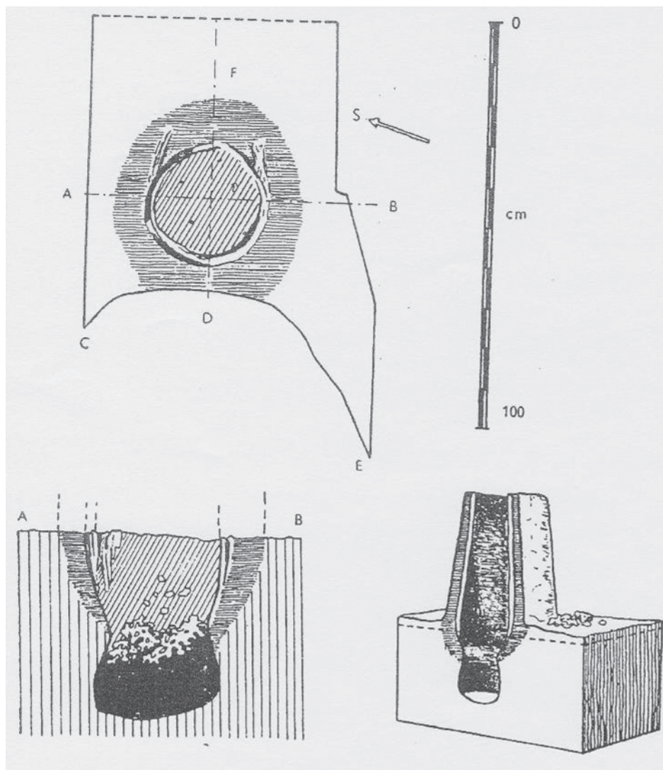
Půdorys a řez germánskou železářskou pecí včetně její rekonstrukce z 1. století n. l. podle nálezu z Luštěnic
